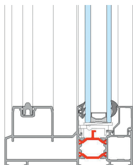
Buiten kader monorail Dormant - monorail
