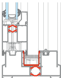
Kader-vleugelcombinatie duorail Dormant-ouvrant duorail
