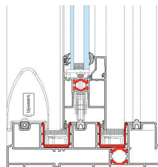
Kader-vleugelcombinatie tri rail Dormant-ouvrant tri rail
