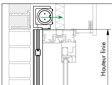
Encastré au-dessus du châssis avec équerres, sans caisson
