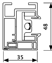
Coulisse ouverte (S+)
