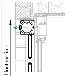
Avant-corps , devant le châssis à l'extérieur
