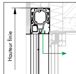
Avant-corps intégré, avec caisson, pour plâtrage
