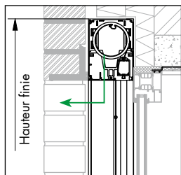
Avant-corps intégré, avec caisson
