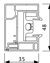
Coulisse fermée (G)
