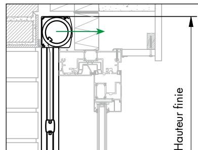
Au-dessus du châssis , avec caisson inversé, sans profil avant
