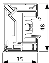
Coulisse fermée (G) M7
