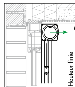
Avant-corps , devant le châssis à l'intérieur
